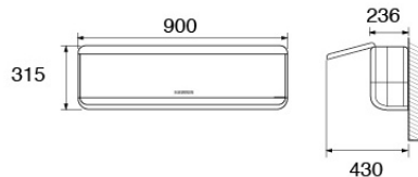
BSI-36KIGSH BSI-41KIGSH BSI-50KIGSH
