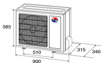
DTE-41K18V DTE-50K20V
