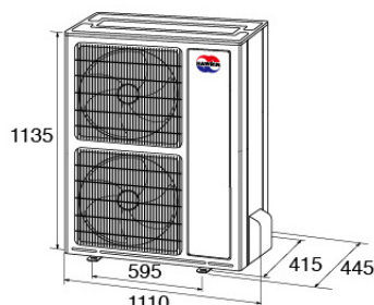
DT-102KVF DT-120KVF
