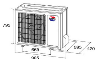
DTS-80K35V
