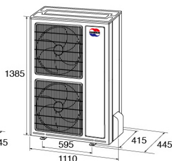
DT-140KVF DT-160KVF
