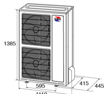
DT-140KVF DT-160KVF
